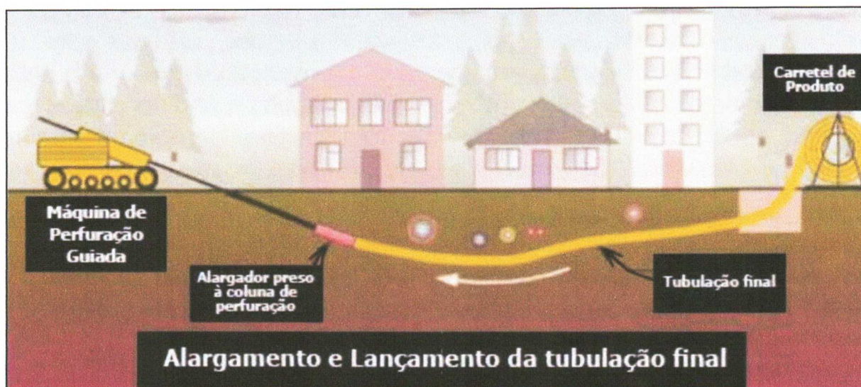
Figura 6 – Ilustração da segunda e terceira etapas da execução
