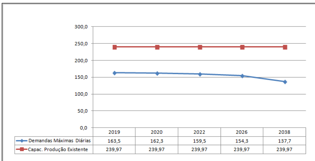
Gráfico 4.6 – Demandas Máximas Diárias (l/s) x Capacidade de Produção (l/s) x Anos de Planejamento
