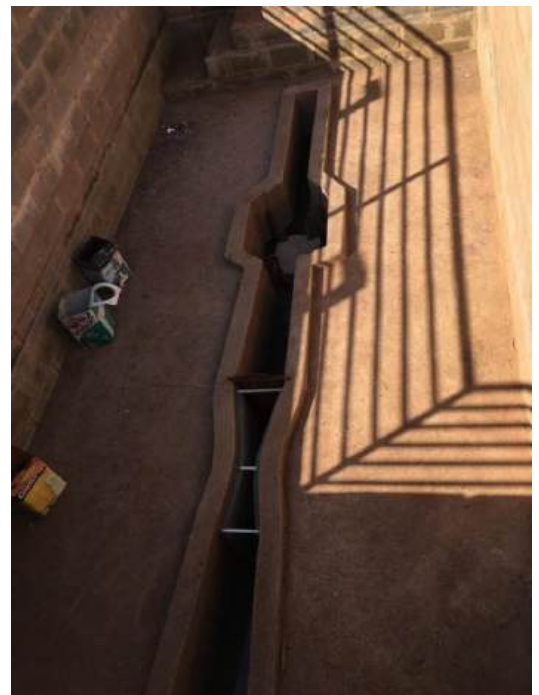
Foto 3.111 – Detalhe da Calha Parshall e do gradeamento
