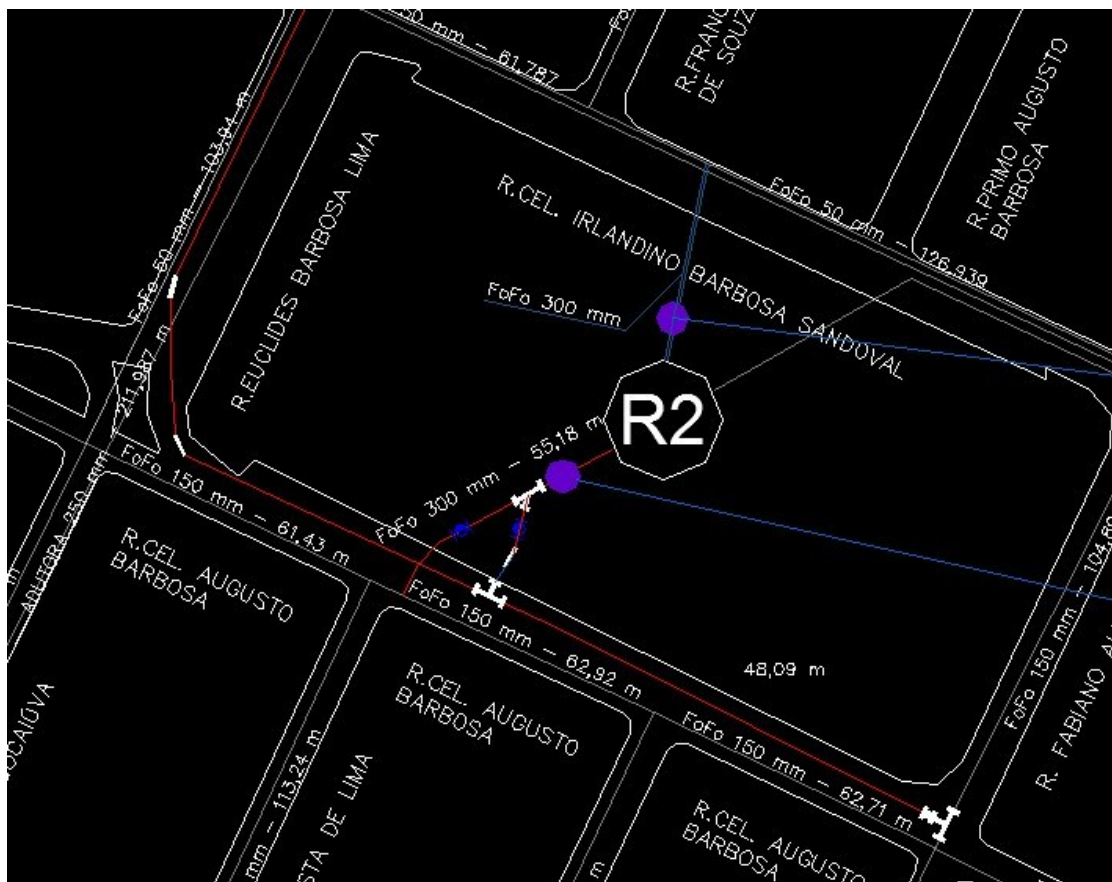
Local de Instalação dos macros medidores.
