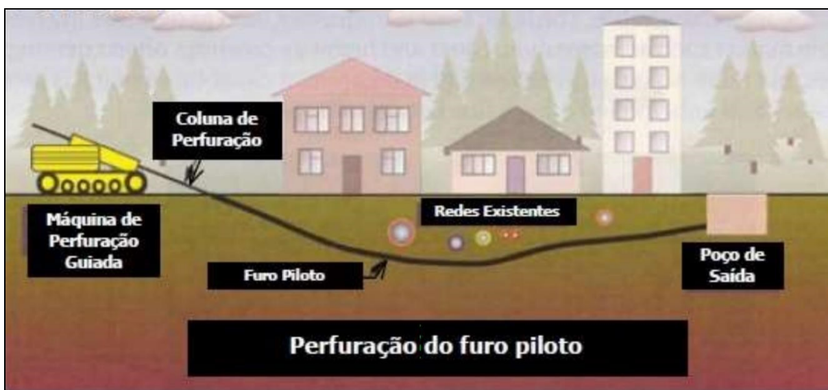
Figura 5 – Ilustração da primeira etapa da execução
