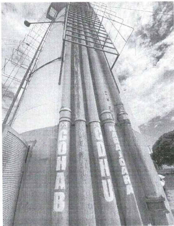
Fotos 04 e 05 – Redes de distribuição para bairros da Central de Reserva da Cohab
