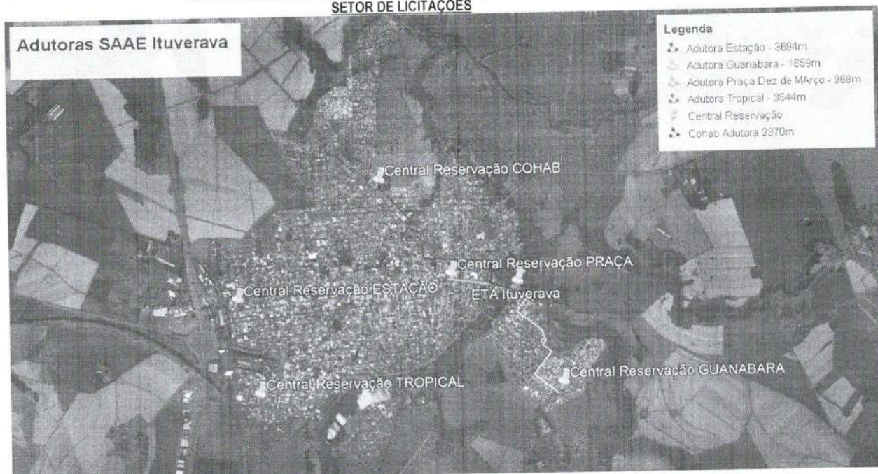
Figura 02 – Rede de Adução e Centrais de Reserva do Sistema de Abastecimento de Água de Ituverava
